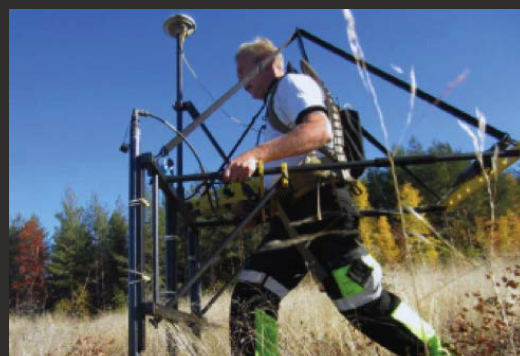
Manuell dataloggning (3 GPS sonder). Lämpar sig för framkomliga kuperade områden.
